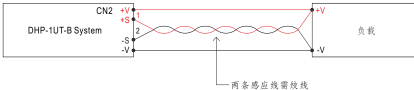
图 1-1 线压降补偿配线示意图
