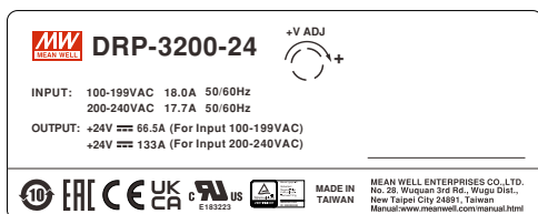
圖1-1 DRP-3200單體標示貼紙
