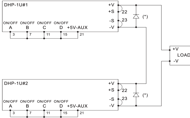
圖3-9 串聯操作配置方式示意圖
