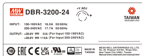
圖1-2 DBR-3200單體標示貼紙
