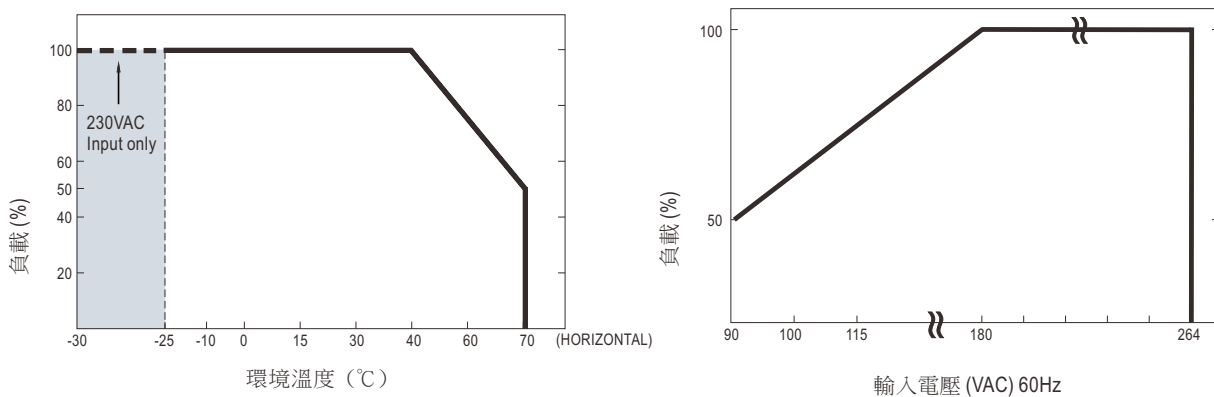
圖5-2 DHP-1U減額曲線
