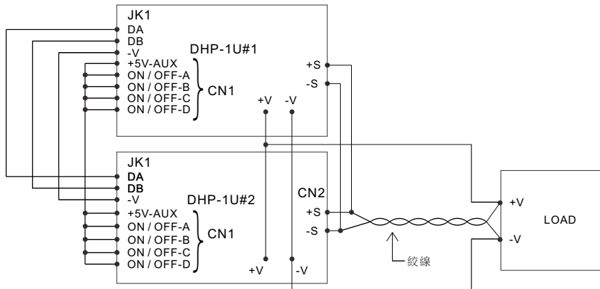
圖3-8 二組整機並聯連接
