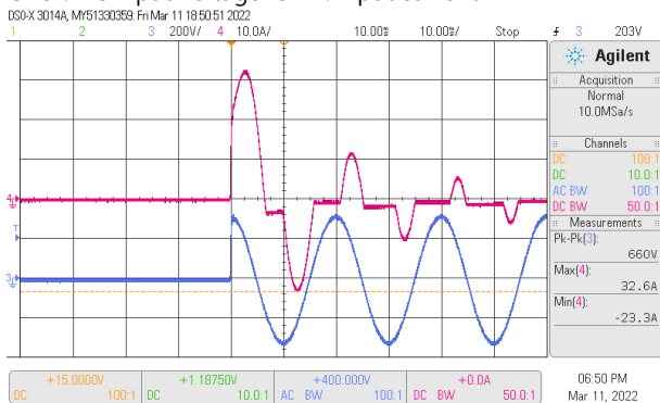
CH3 : AC Input Voltage CH4 : Input current
